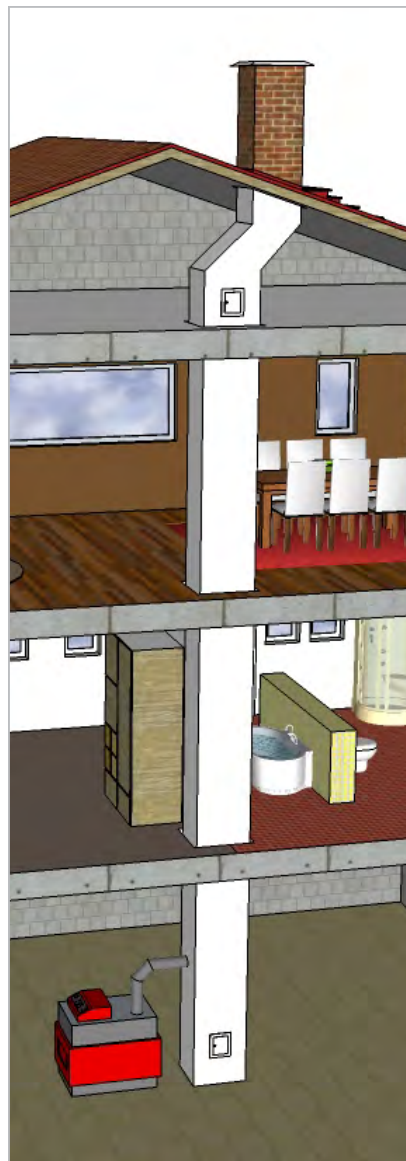
gezogener und gerader Schornstein mit 2. Reinigung unterhalb des Daches
