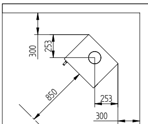
Avstand til brennbart materiale uten isolert røykrør
