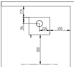
Avstånd till brännbart material utan isolerat röktör
