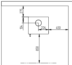
Abstand zu brennbarem Material ohne isoliertes Rauchrohr
