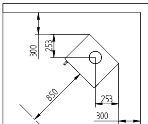
Abstand zu brennbarem Material ohne isoliertes Rauchrohr
