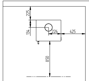
Avstånd till brännbart material med isolerat röktör
