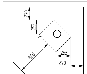
Avstånd till brännbart material med isolerat röktör
