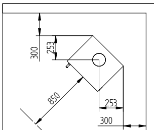
Avstånd till brännbart material utan isolerat röktör
