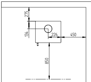
Avstand til brennbart materiale uten isolert røykrør
