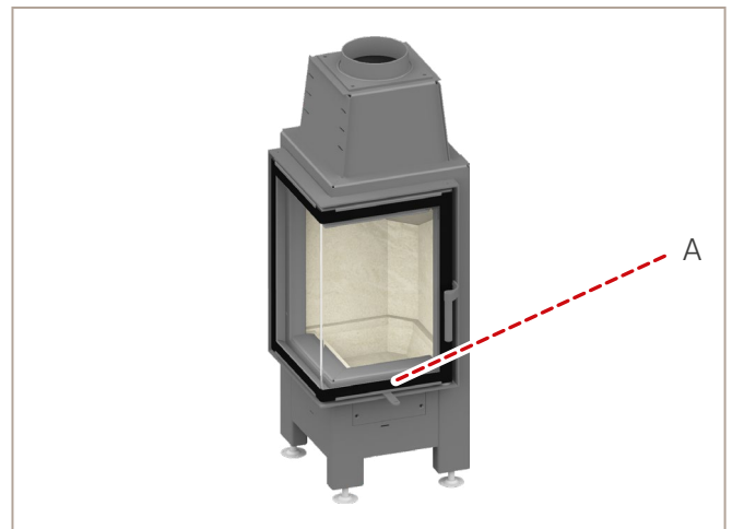
Abb. 30: Rostlose Verbrennung (mit Bodensteinen) am Beispiel Ekko 34(34)51 s
