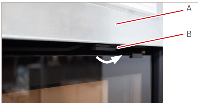
Abb. 31: Schließzunge Front geschlossen
