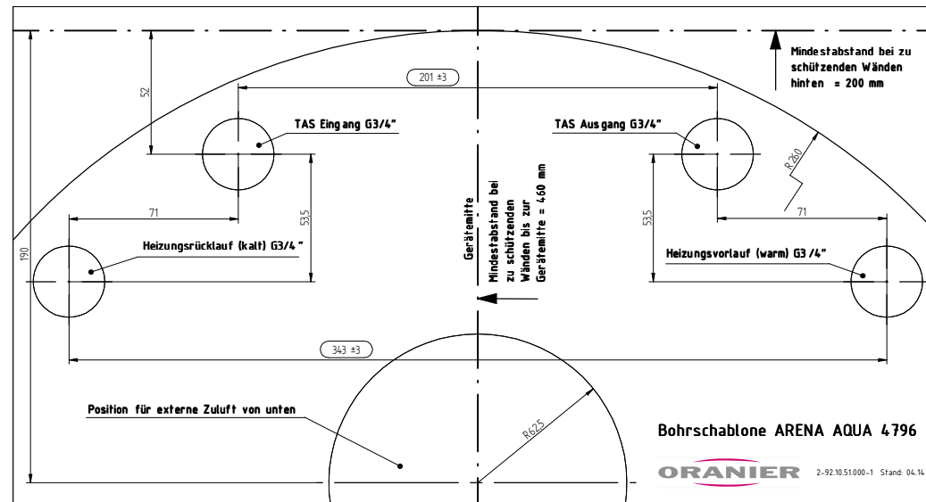
Darstellung der bedruckten Schablone
