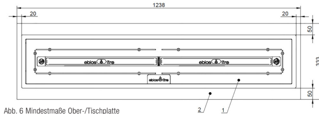
Abb. 6 Mindestmaße Ober-/Tischplatte
