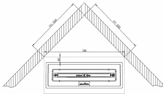
Abb. 14 Mindestabstände in einer Raumecke
