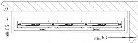
Abb. 21 Mindestabstände zur Wand
