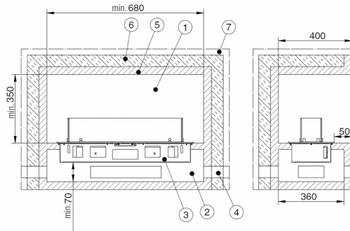
Abb. 28 Mindestmaße Feuerraum
