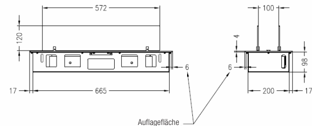
Abbildung Quadra Inside I SL:
