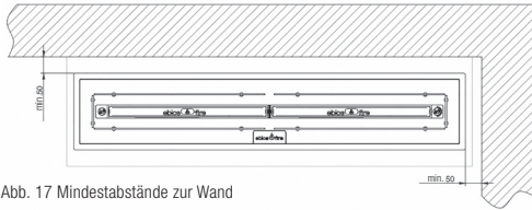
Abb. 17 Mindestabstände zur Wand
