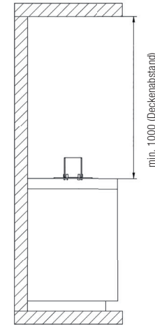
Abb. 15 Mindestabstand Deckel
