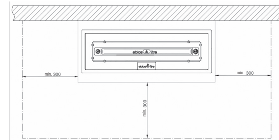
Abb. 16 Mindestabstände zu brennbaren Bauteilen
