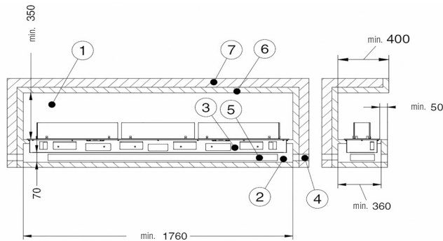
Abb. 30 Mindestmaße Feuerraum
