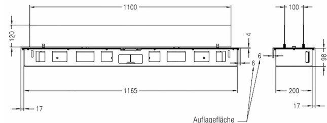
Abbildung Quadra Inside II SL:
