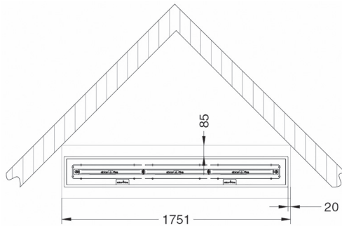
Abb. 22 Mindestabstände in einer Raumecke
