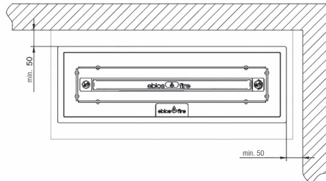
Abb. 13 Mindestabstände zur Wand
