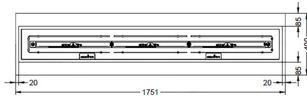
Abb. 8 Mindestmaße Ober-/Tischplatte
