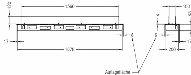
Abbildung Quadra Inside III SL:
