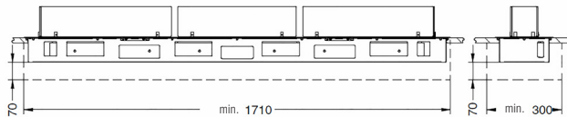
Abb. 5 Mindestmaße Gehäuseraum
