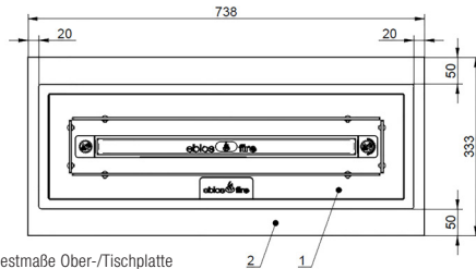
Abb. 4 Mindestmaße Ober-/Tischplatte
