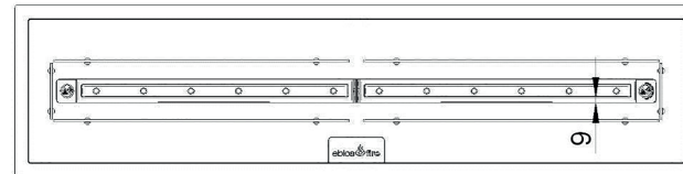
Abb. 11 Luftspalt ca. 9 mm (ohne Abdeckblech)
