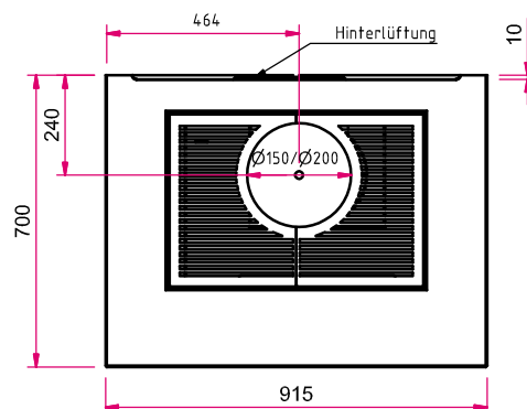
Draufsicht M 1:20
