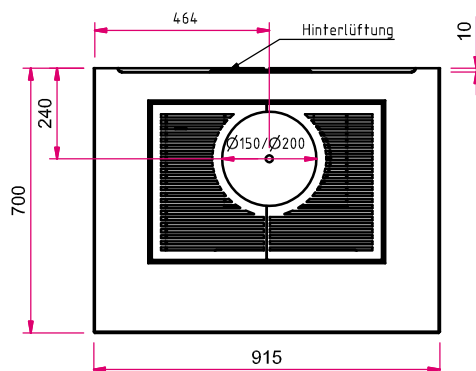
Draufsicht M 1:20
