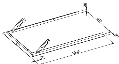
Tragrahmen: SERA 55 US (1004-00765)
