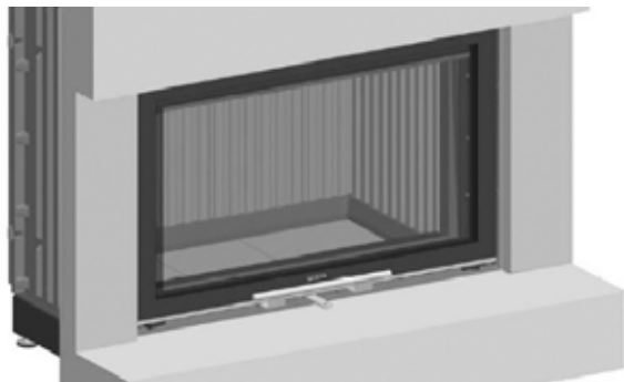
SERA ohne Blenden: Einbaubeispiel
