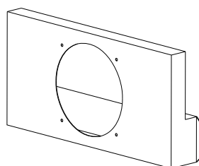
Verbrennungsluft-Anschlusskasten (1004-00574)
