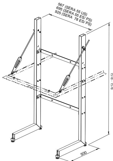
Variables Traggestell: ohne Tragrahmen (1004-00768/ 1004-00681)
